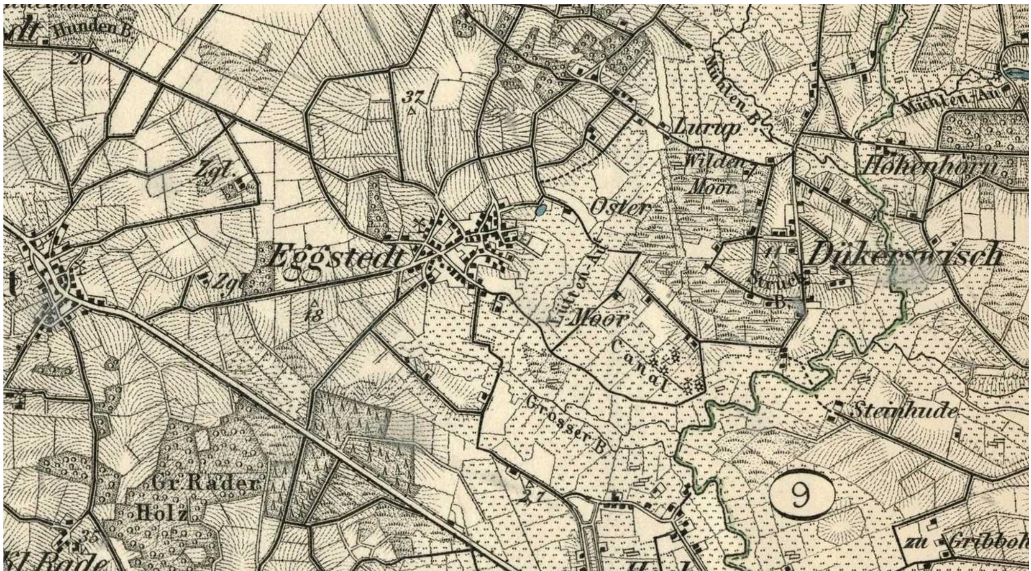
Auszug Eggstedt aus der TK25 Jahrgang 1880 – Süderhastedt 1921
